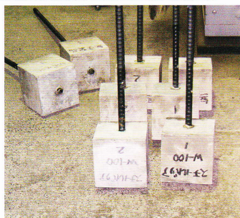
附着強度試験被検体
